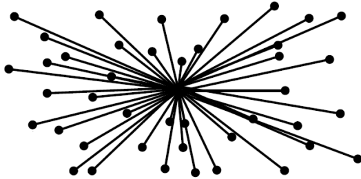
Centralistic PKI
